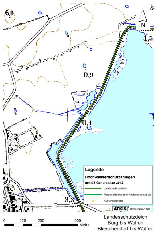
Abb. 313: Lageplan Landesschutzdeich Burg bis Wulfen (Blieschendorf bis Wulfen)LKN-SH 2011
