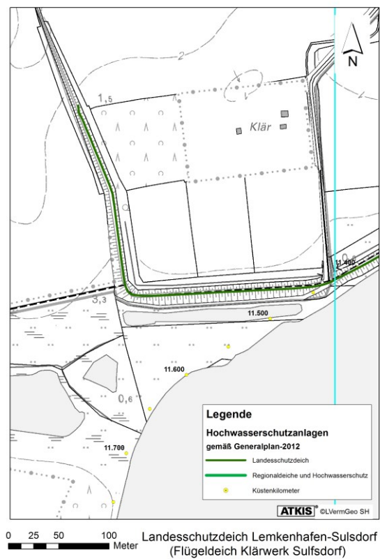
Abb. 91: Lageplan des Landesschutzdeiches Lemkenhafen-Sulsdorf (Flügeldeich Klärwerk Sulsdorf) LKN-SH 2011
