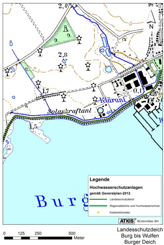
Abb. 299: Lageplan Landesschutzdeich Burg bis Wulfen (Burger Deich)LKN-SH 2011
