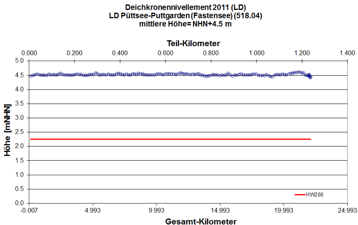
Abb. 182: Längsprofil Landesschutzdeich Püttsee-Puttgarden (Fastensee) Deichkronennivellement 2011 LKN-SH 2011
