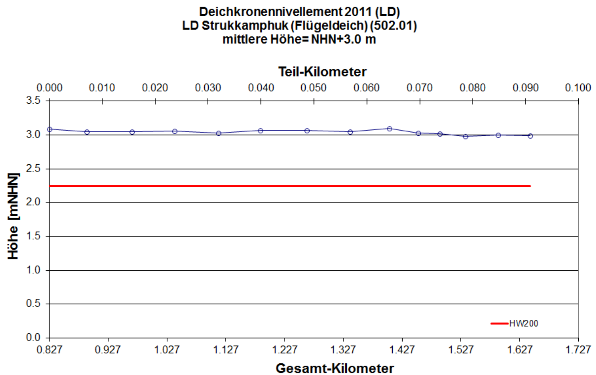
Abb. 5: Längsprofil des Landesschutzdeiches Struckkamphuk (Flügeldeich) Deichkronennivellement 2011 LKN-SH 2011
