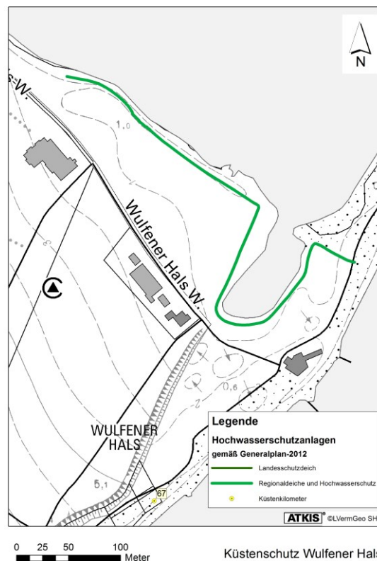
Abb. 333: Lageplan Küstenschutz Wulfener Hals (Golfplatz) LKN-SH 2011
