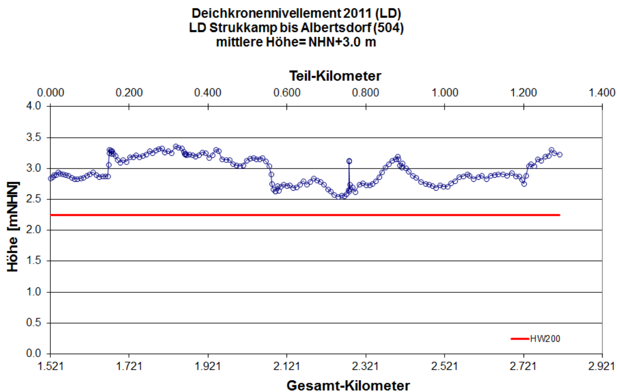
Abb. 20: Längsprofil des Landesschutzdeiches Struckamp bis Albertsdorf Deichkronennivellement 2011 LKN-SH 2011
