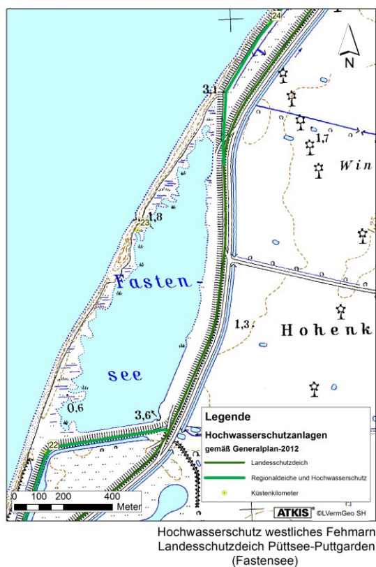
Abb. 181: Lageplan Landesschutzdeich Püttsee-Puttgarden (Fastensee) LKN-SH 2011
