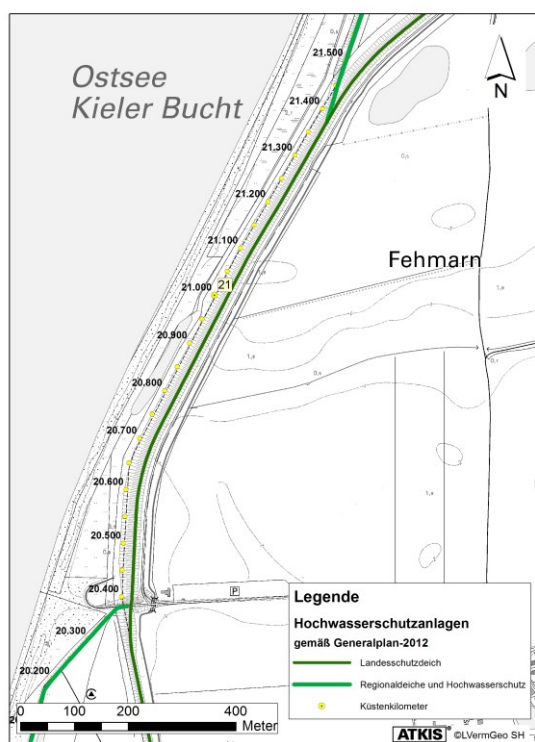
Hochwasserschutz westliches Fehmarn Landesschutzdeich Püttsee-Puttgarden (Bojendorfer Strandweg bis südlich Deichrückverlegung Fastensee)
