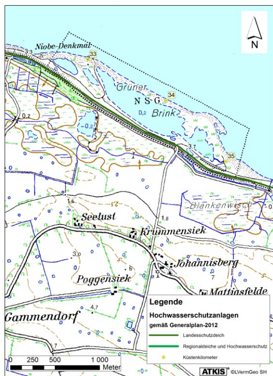
Hochwasserschutz westliches Fehmarn Landesschutzdeich Püttsee-Püttgarden (Grüner Brink)
