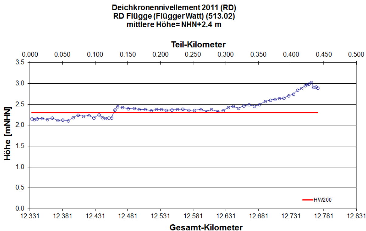
Abb. 109: Längsprofil des Regionaldeiches Flügge (Flügger Watt) Deichkronennivellement 2011 LKN-SH 2011
