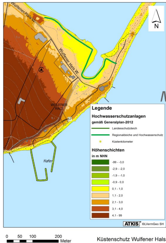
Abb. 334: Geländehöhen im Bereich Wulfener Hals (Golfplatz) LKN-SH 2015
