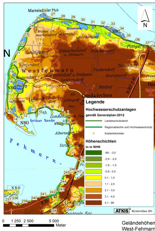
Abb. 147: Geländehöhen im westlichen Teil Fehmarns LKN-SH 2015
