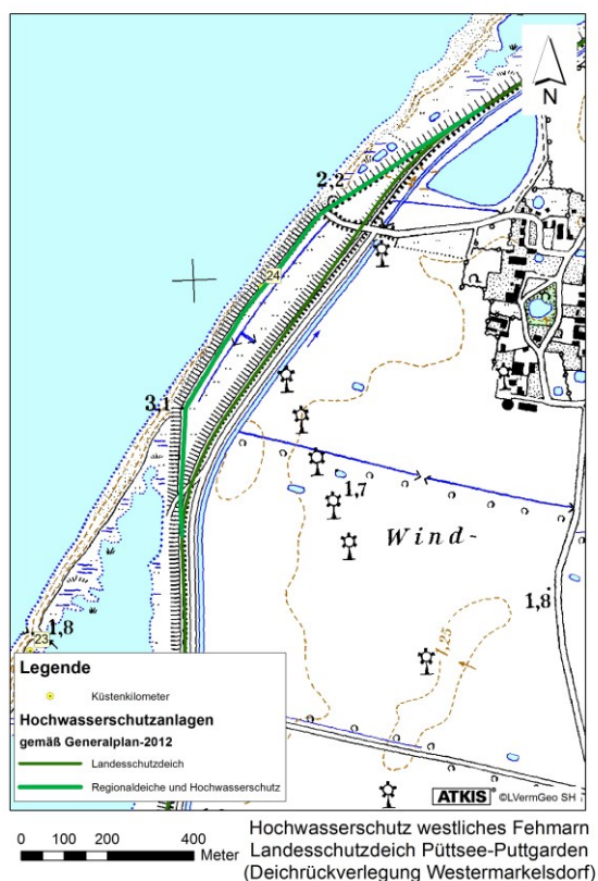
Abb. 191: Lageplan Landesschutzdeich Püttsee-Püttgarden (Deichrückverlegung Westermarkelsdorf) LKN-SH 2011
