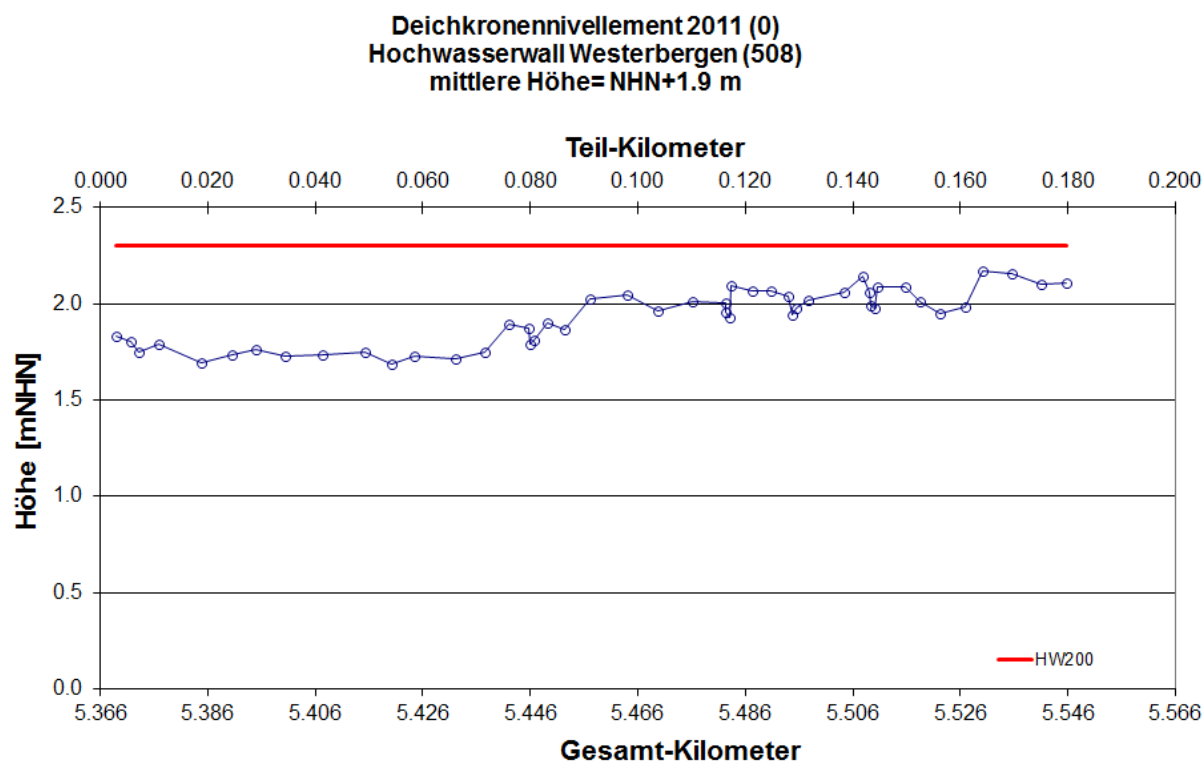
Abb. 47: Längsprofil des Hochwasserschutzes Westerbergen 2011 LKN-SH 2011
