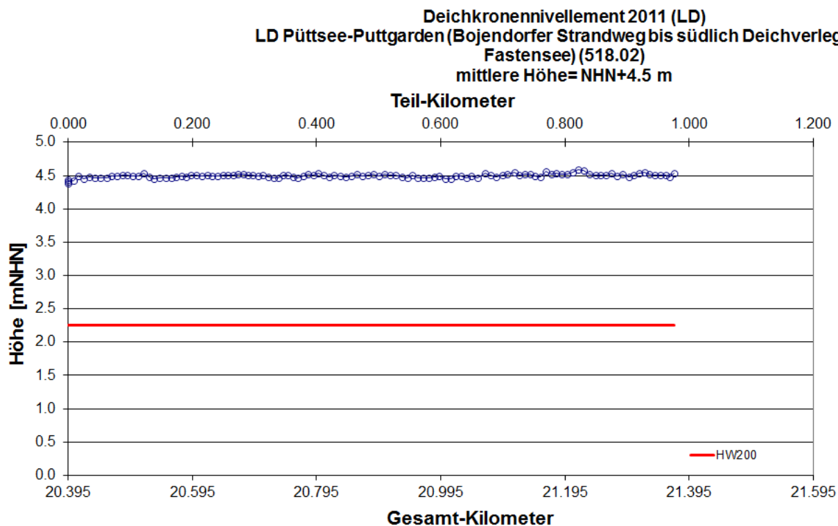
Abb. 167: Längsprofil Landesschutzdeich Püttsee-Puttgarden (Bojendorfer Strandweg bis südlich Deichrückverlegung Fastensee) Deichkronennivellement 2011 LKN-SH 2011
