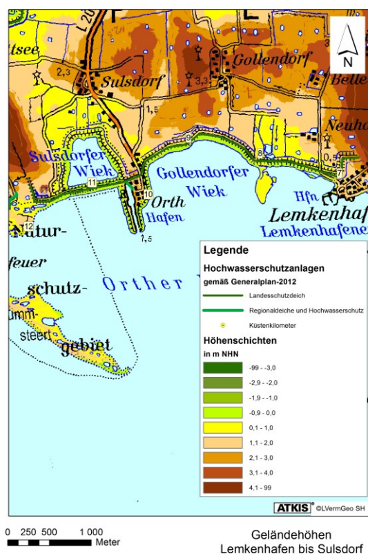
Abb. 53: Geländehöhen im Bereich Lemkenhafen bis Suldsdorf LKN-SH 2015
