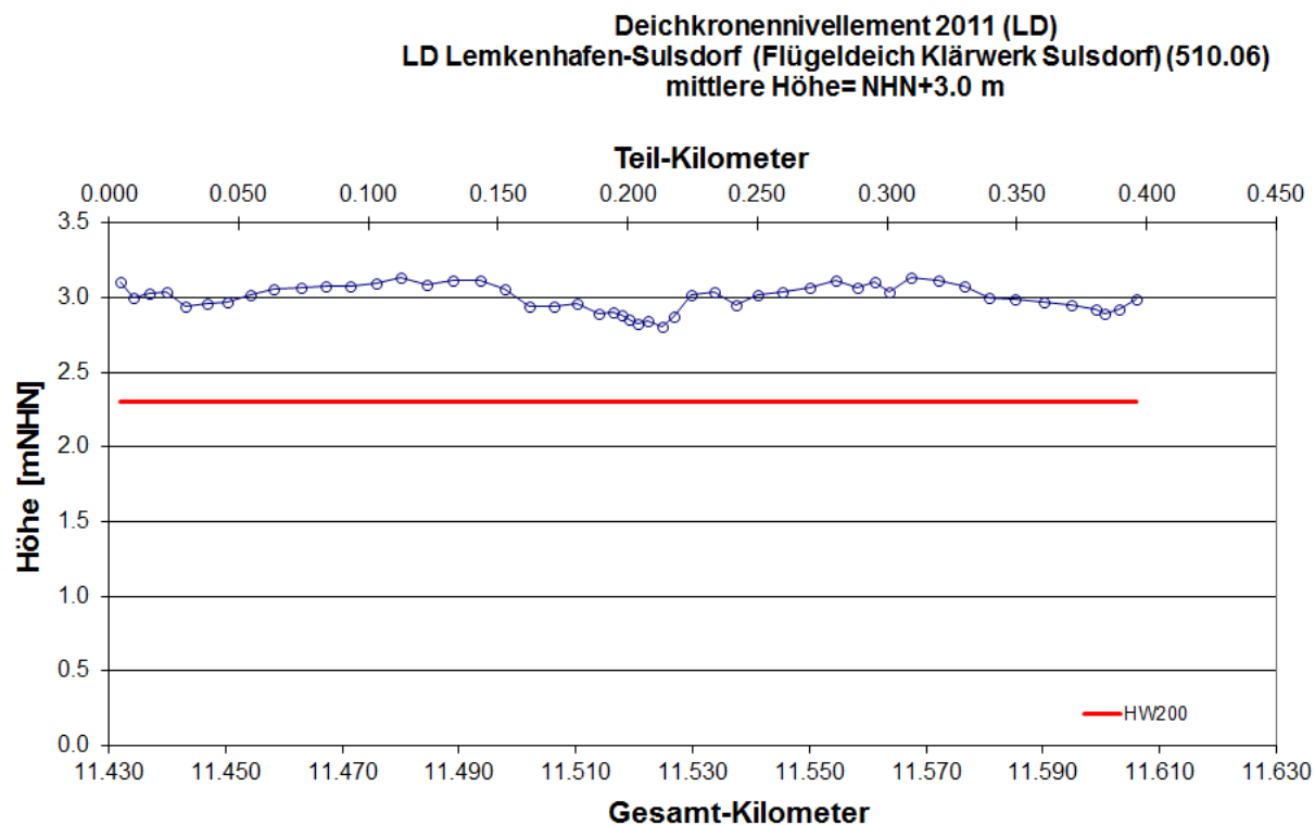
Abb. 92: Längsprofil des Landesschutzdeiches Lemkenhafen-Sulsdorf (Flügeldeich Klärwerk Sulsdorf)) Deichkronennivellement 2011 LKN-SH 2011
