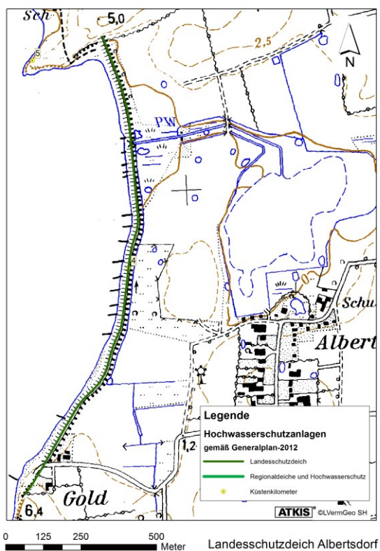
Abb. 34: Lageplan des Landesschutzdeiches Albertsdorf LKN-SH 2011
