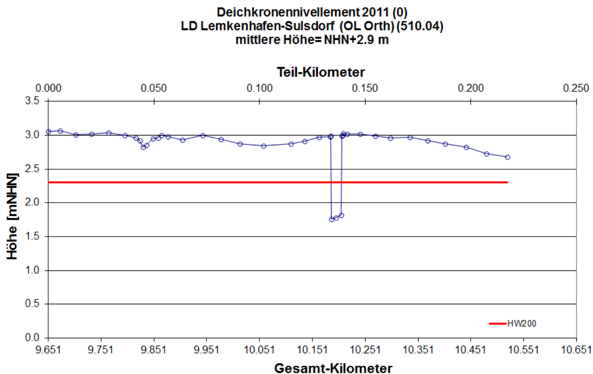
Abb. 77: Längsprofil des Landesschutzdeiches Lemkenhafen-Sulsdorf (OL Orth) Deichkronennivellement 2011 LKN-SH 2011
