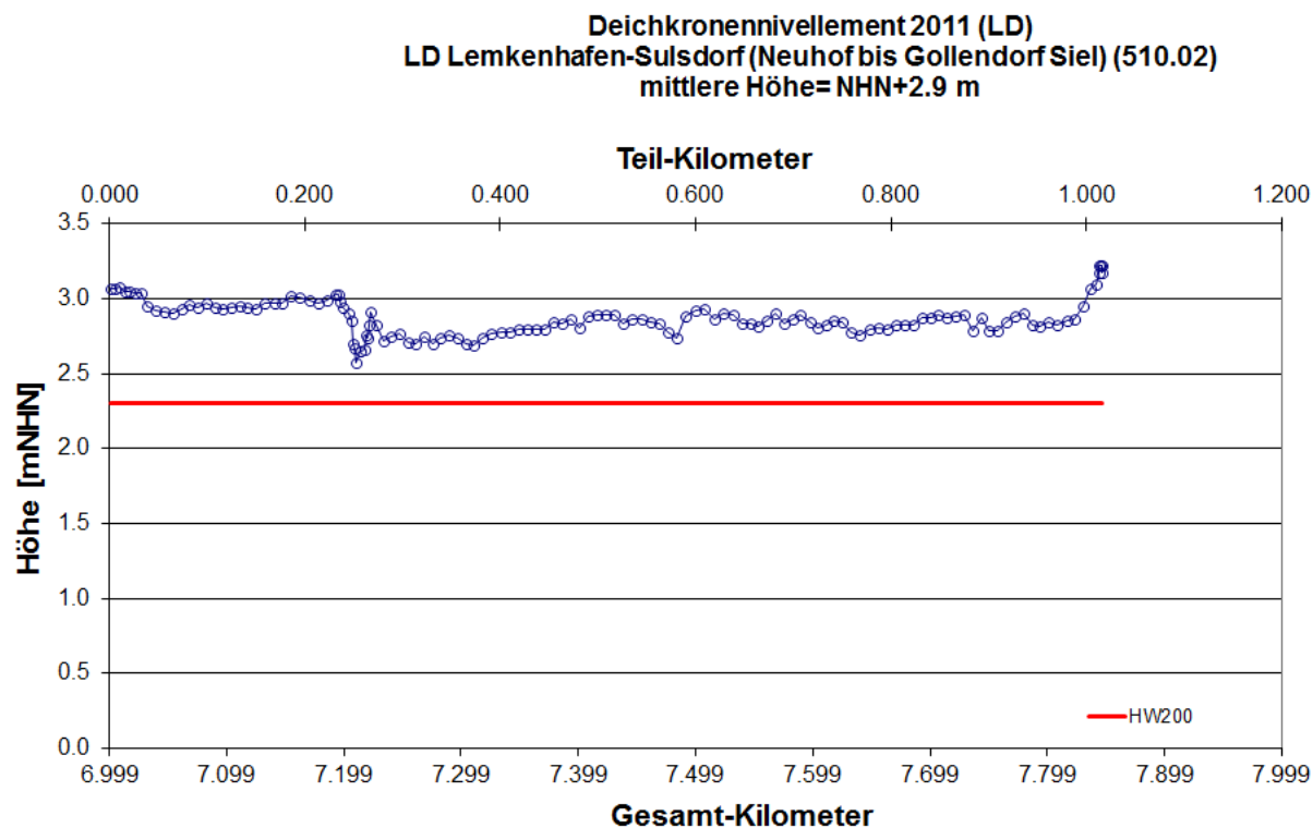
Abb. 60: Längsprofil des Landesschutzdeiches Lemkenhafen-Sulsdorf (Neuhof bis Gollendorf Siel) Deichkronennivellement 2011 LKN-SH 2011
