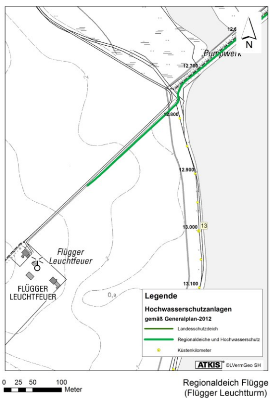
Abb. 116: Lageplan des Regionaldeiches Flügge (Flügger Leuchtturm) LKN-SH 2011
