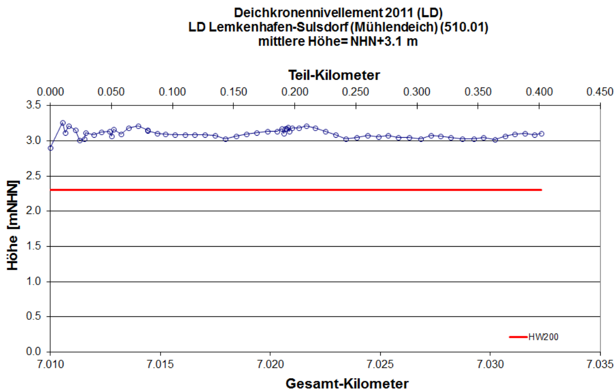
Abb. 55: Längsprofil des Landesschutzdeiches Lemkenhafen-Sulsdorf (Mühlendeich) Deichkronennivellement 2011 LKN-SH 2011
