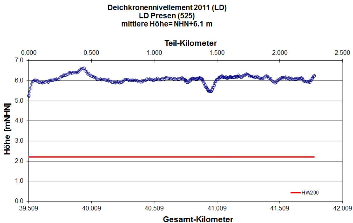
Abb. 275: Längsprofil Landesschutzdeich Presen Deichkronennivellement 2011 LKN-SH 2011
