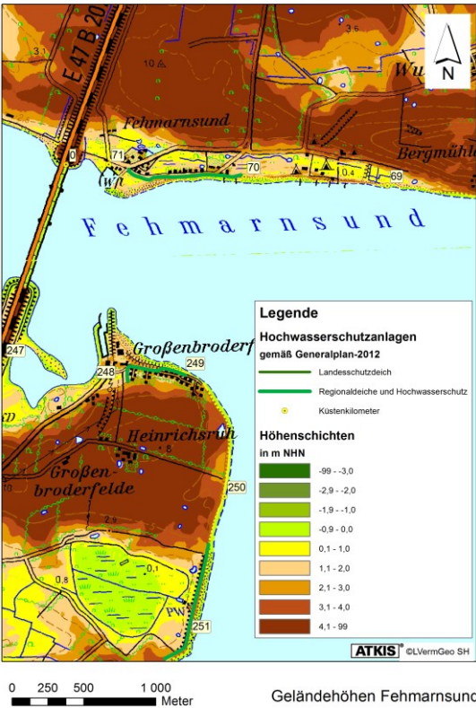
Abb. 342: Geländehöhen im Bereich Fehmarnsund LKN-SH 2015
