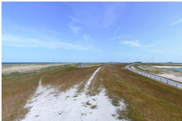
Abb. 177: Deich, Krone und Böschungen bei rd. Kkm 21,39, Blickrichtung Nord LKN-SH 2004-06-01_01542 Juni 2004
