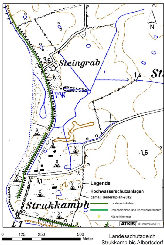
Abb. 19: Lageplan des Landesschutzdeiches Strukkamp bis Albertsdorf LKN-SH 2011
