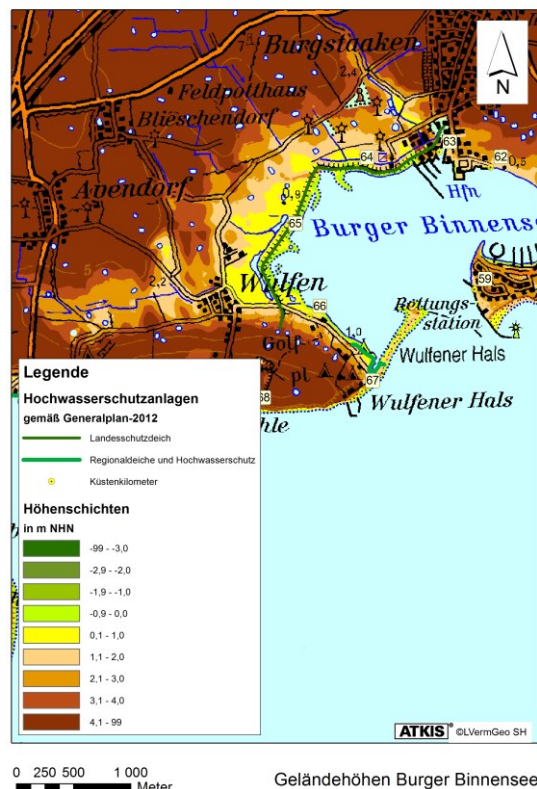
Abb. 288: Geländehöhen im Bereich des westlichen Burger Binnensees LKN-SH 2015
