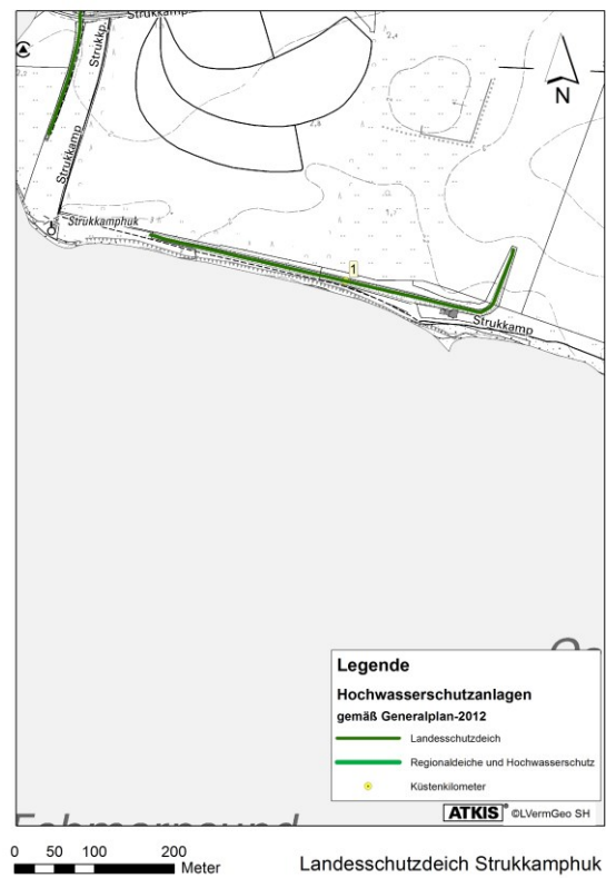
Abb. 4: Lageplan des Landesschutzdeiches Struckamphuk LKN-SH 2011
