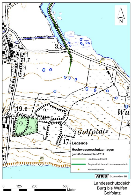
Abb. 326: Lageplan Landesschutzdeich Burg bis Wulfen (Golfplatz) LKN-SH 2011
