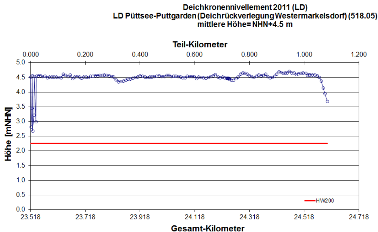
Abb. 192: Längsprofil Landesschutzdeich Püttsee-Puttgarden (Deichrückverlegung Westermarkelsdorf) Deichkronennivellement 2011 LKN-SH 2011
