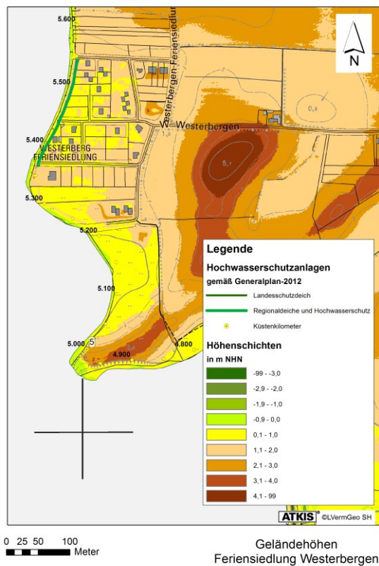
Abb. 45: Geländehöhen im Bereich Feriensiedlung Westerbergen LKN-SH 2015
