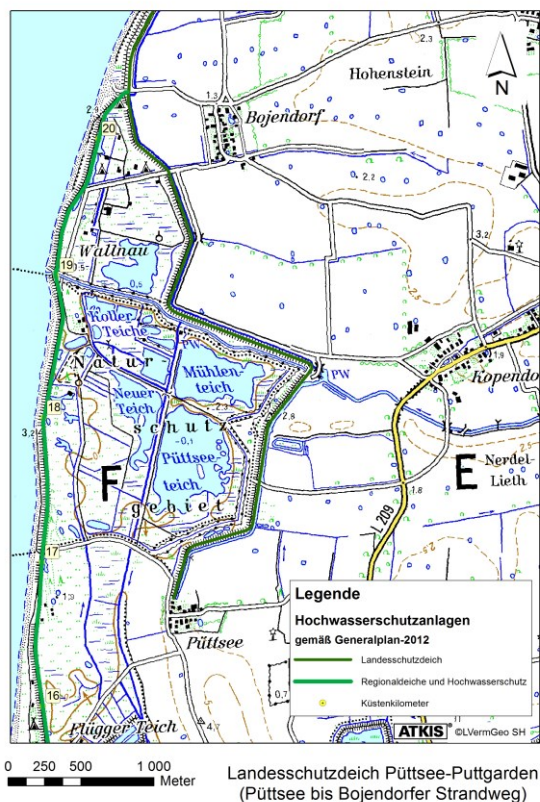
Abb. 149: Lageplan Landesschutzdeich Püttsee-Puttgarden (Püttsee bis Bojendorfer Strandweg) LKN-SH 2011
