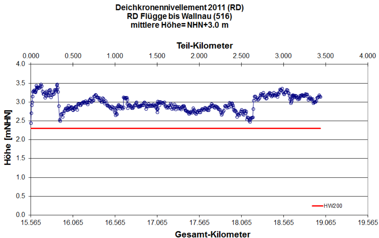
Abb. 123: Längsprofil des Regionaldeiches Flügge bis Wallnau Deichkronennivellement 2011 LKN-SH 2011
