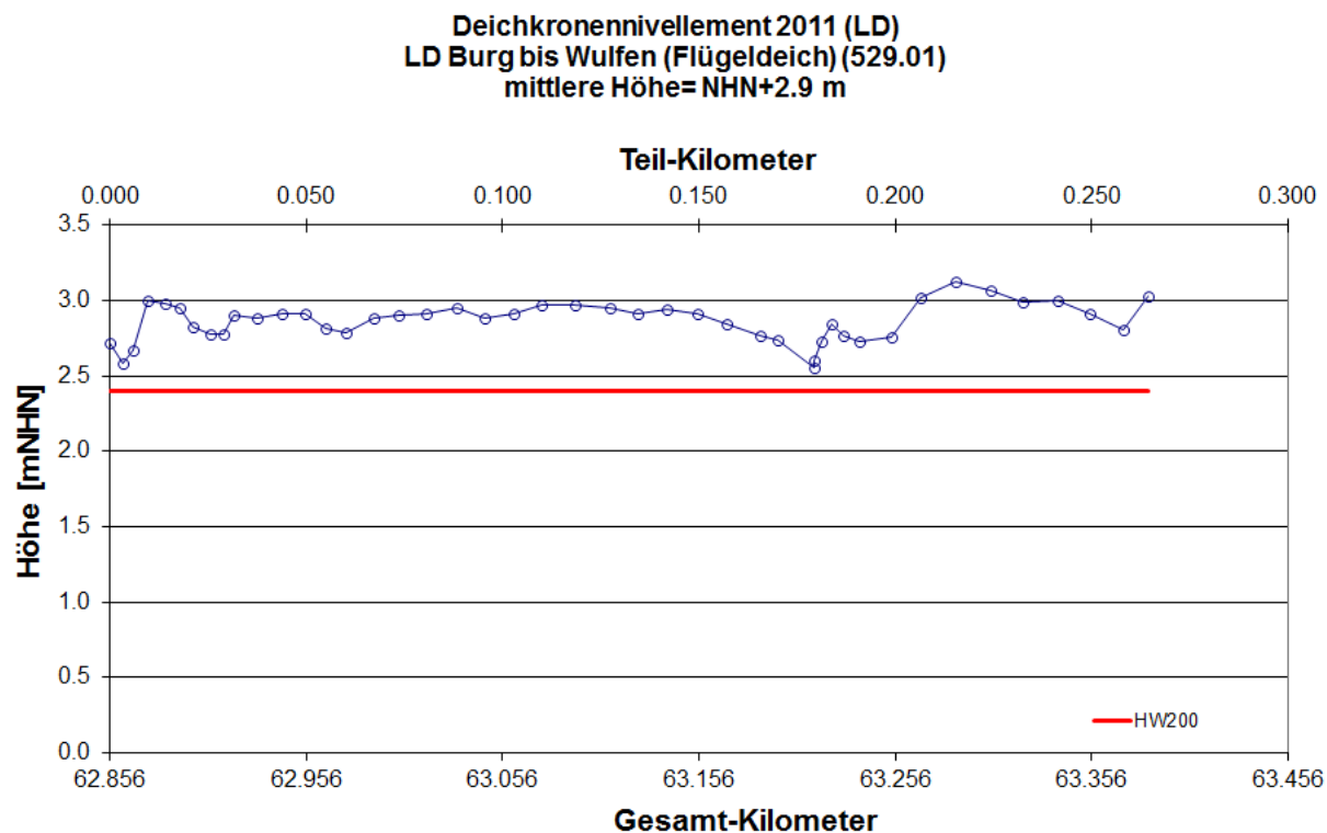
Abb. 291: Längsprofil Landesschutzdeich Burg bis Wulfen (Flügeldeich) Deichkronennivellement 2011 LKN-SH 2011
