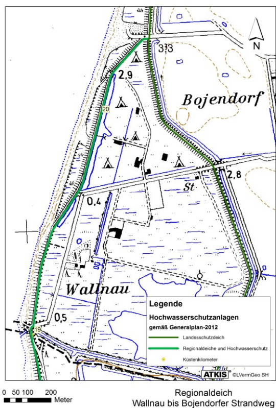
Abb. 136: Lageplan des Regionaldeiches Flügge bis Wallnau LKN-SH 2011
