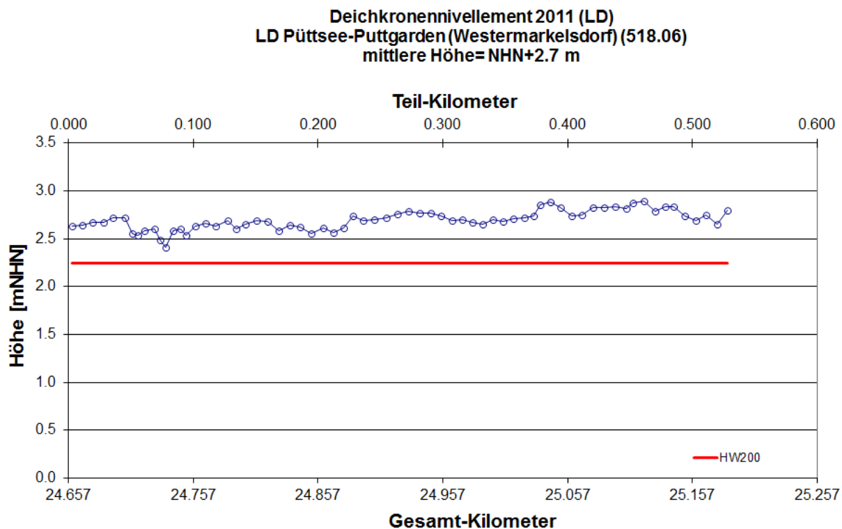
Abb. 202: Längsprofil Landesschutzdeich Püttsee-Puttgarden (Westermarkelsdorf) Deichkronennivellement 2011 LKN-SH 2011
