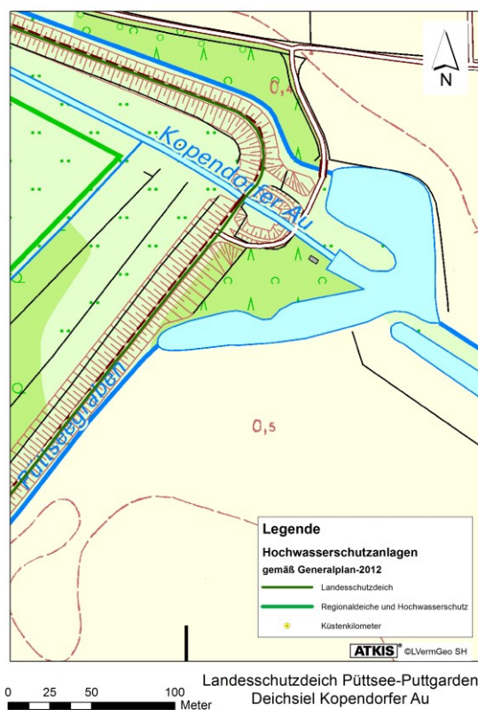
Abb. 156: Deichsiel Kopendorfer Au bei rd. Kkm 18,40, Lageplan Nord LKN-SH 2016
