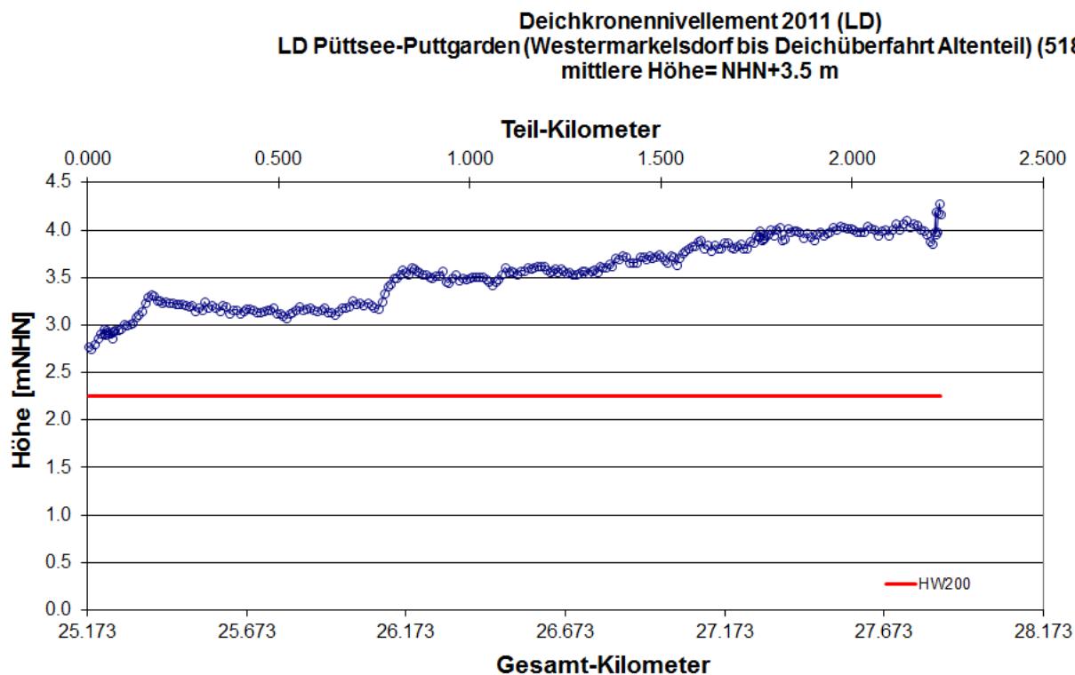
Abb. 209: Längsprofil Landesschutzdeich Püttsee-Puttgarden (Westermarkelsdorf bis Deichüberfahrt Altenteil) Deichkronennivellement 2011 LKN-SH 2011
