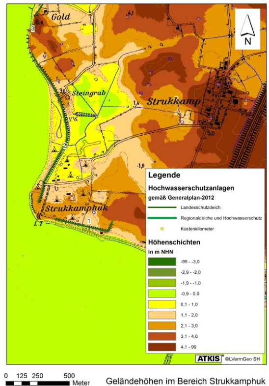
Abb. 3: Geländehöhen im Bereich Strukkamphuk LKN-SH 2015
