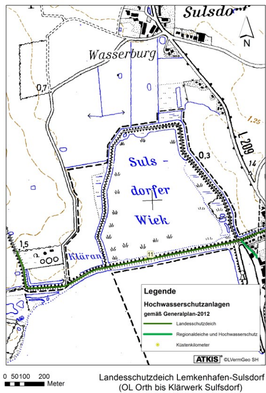
Abb. 83: Lageplan des Landesschutzdeiches Lemkenhafen-Sulsdorf (OL Orth bis Klärwerk Sulfsdorf) LKN-SH 2011
