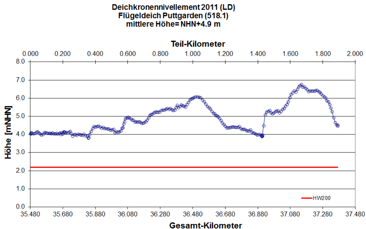
Abb. 259: Längsprofil Landesschutzdeich Püttsee-Puttgarden (Puttgarden) Deichkronennivellement 2011 LKN-SH 2011
