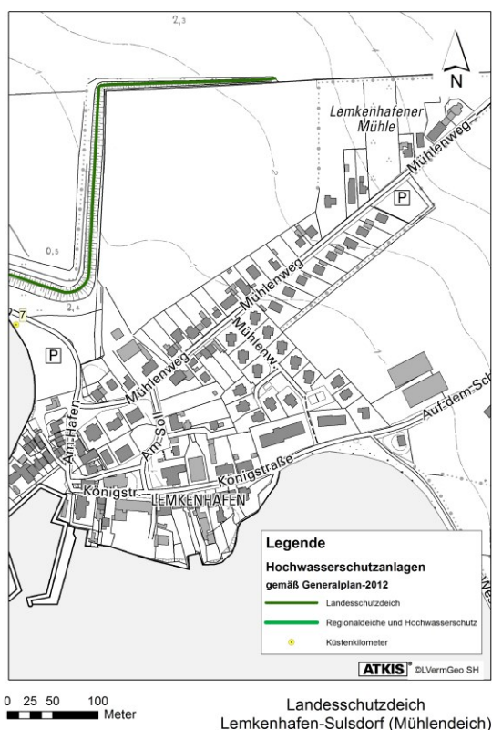
Abb. 54: Lageplan des Landesschutzdeiches Lemkenhafen-Sulsdorf (Mühlendeich) LKN-SH 2011
