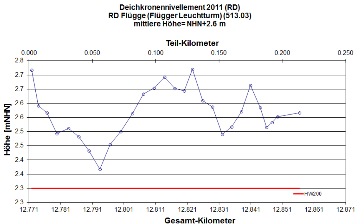
Abb. 117: Längsprofil des Regionaldeiches Flügge (Flügger Leuchtturm) Deichkronennivellement 2011 LKN-SH 2011
