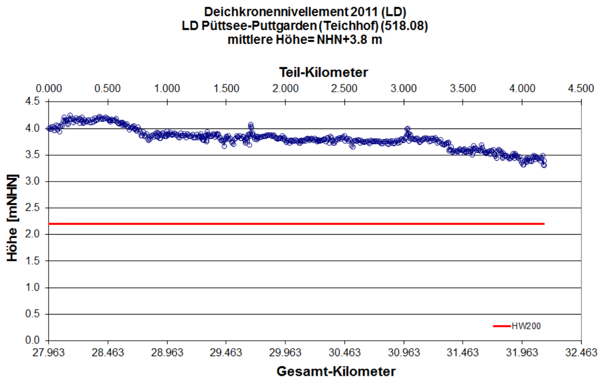
Abb. 222: Längsprofil Landesschutzdeich Püttsee-Puttgarden (Teichhof) Deichkronennivellement 2011 LKN-SH 2011
