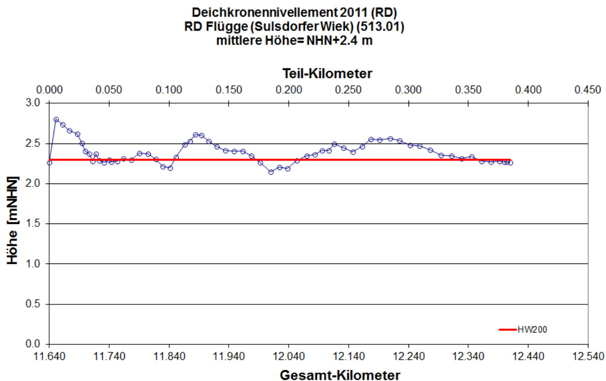
Abb. 102: Längsprofil des Regionaldeiches Flügge (Sulsdorfer Wiek) Deichkronennivellement 2011 LKN-SH 2011
