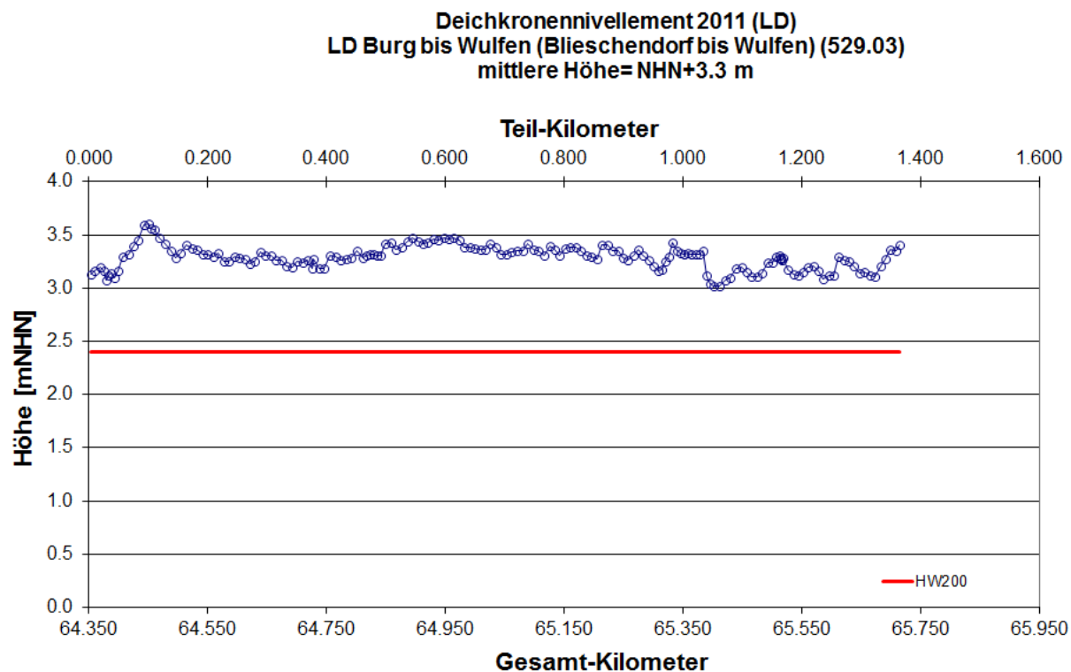
Abb. 314: Längsprofil Landesschutzdeich Burg bis Wulfen (Blieschendorf bis Wulfen) Deichkronennivellement 2011 LKN-SH 2011
