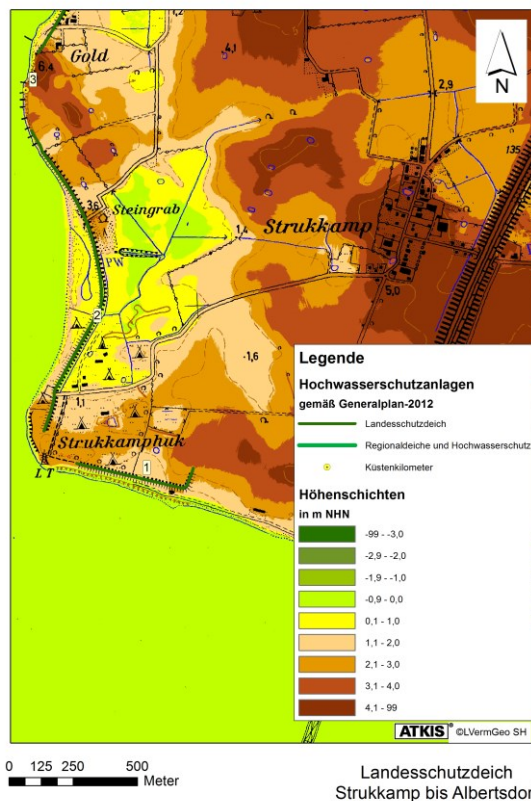
Abb. 18: Geländehöhen im Bereich Strukkamp bis Albertsdorf LKN-SH 2015
