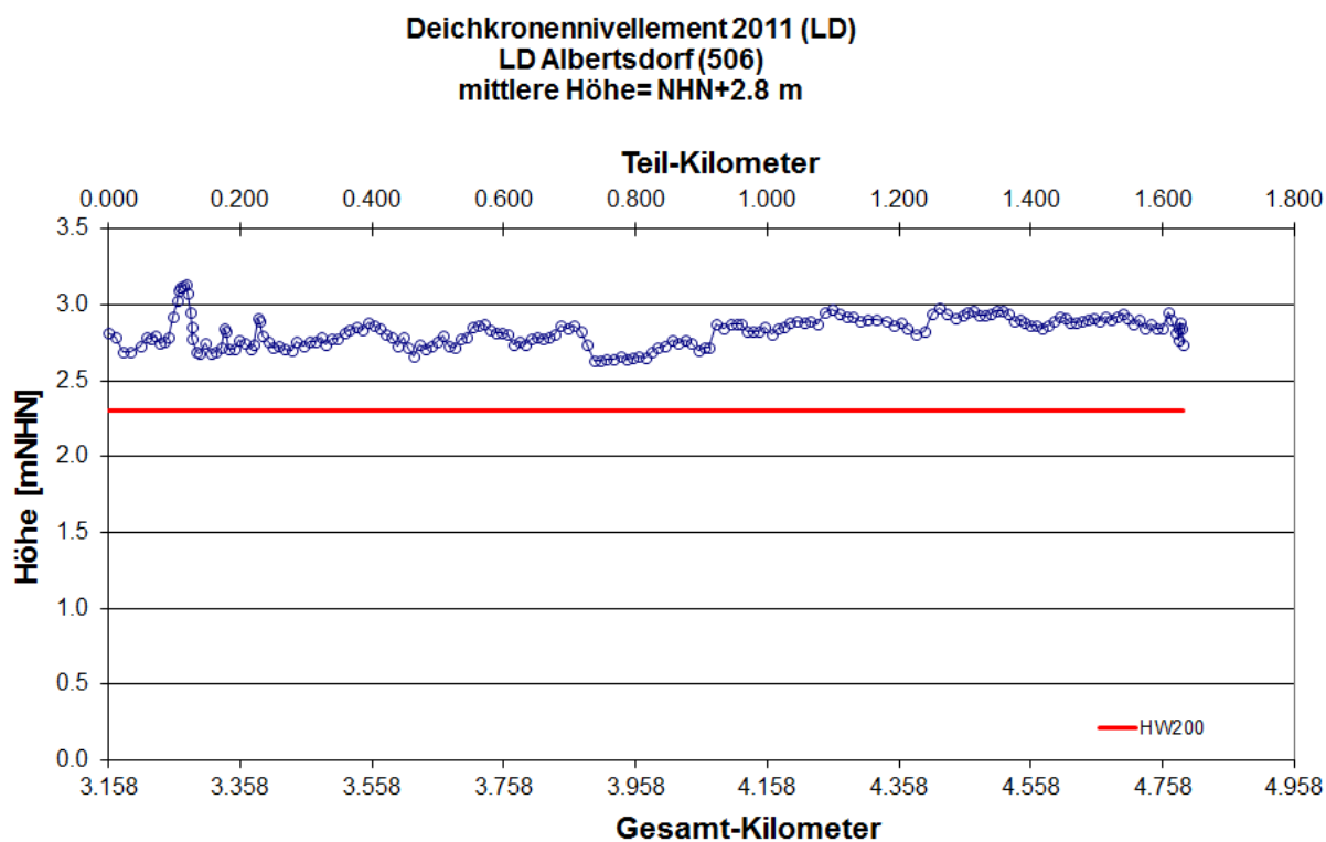
Abb. 35: Längsprofil des Landesschutzdeiches Albertsdorf Deichkronennivellement 2011 LKN-SH 2011
