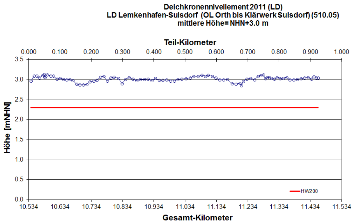
Abb. 84: Längsprofil des Landesschutzdeiches Lemkenhafen-Sulsdorf (OL Orth bis Klärwerk Sulsdorf) Deichkronennivellement 2011 LKN-SH 2011
