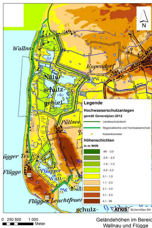
Abb. 98: Geländehöhen im Bereich Flügge und Wallnau LKN-2013
