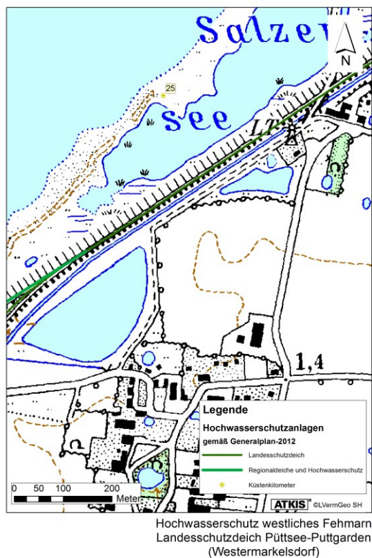
Abb. 201: Lageplan Landesschutzdeich Püttsee-Püttgarden (Westermarkelsdorf) LKN-SH 2011
