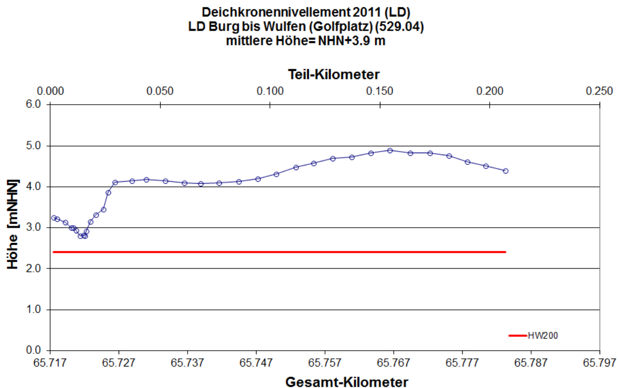
Abb. 327: Längsprofil Landesschutzdeich Burg bis Wulfen (Golfplatz) Deichkronennivellement 2011 LKN-SH 2011
