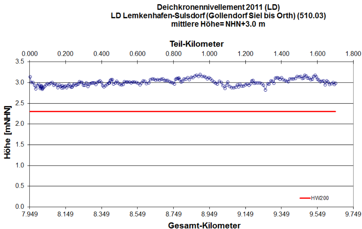
Abb. 69: Längsprofil des Landesschutzdeiches Lemkenhafen-Sulsdorf (Gollendorf Siel bis Orth) Deichkronennivellement 2011 LKN-SH 2011
