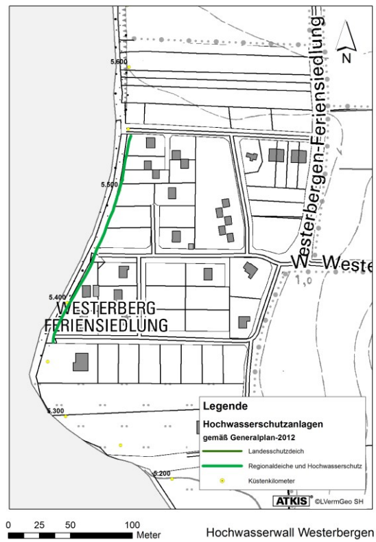
Abb. 46: Lageplan des Hochwasserschutzes Westerbergen LKN-SH 2011
