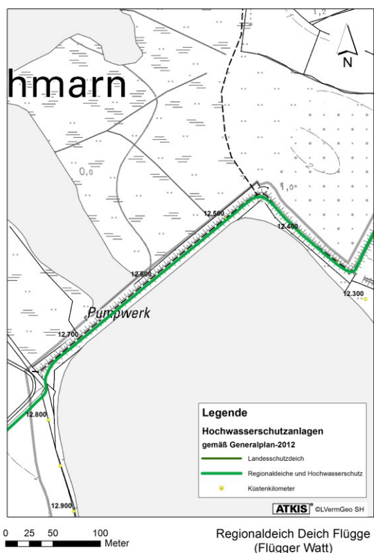
Abb. 108: Lageplan des Regionaldeiches Flügge (Flügger Watt) LKN-SH 2011
