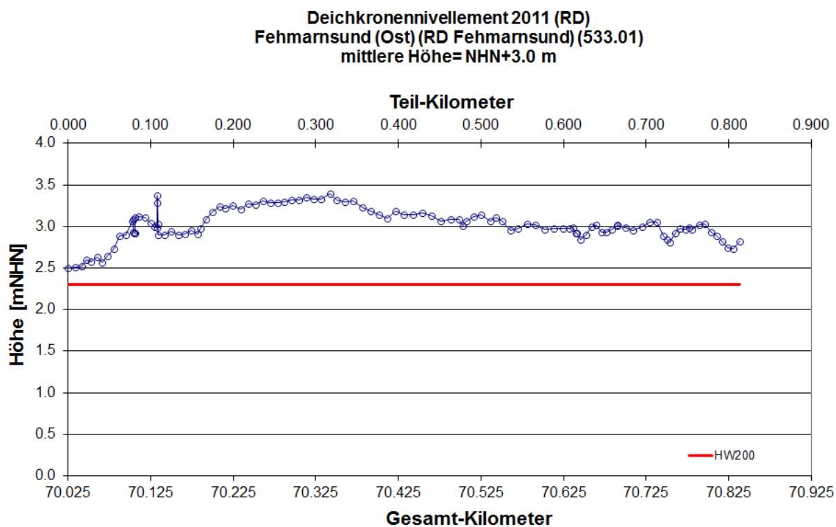
Abb. 344: Längsprofil Regionaldeich Fehmarnsund (Ost) Deichkronennivellement 2011 LKN-SH 2011
