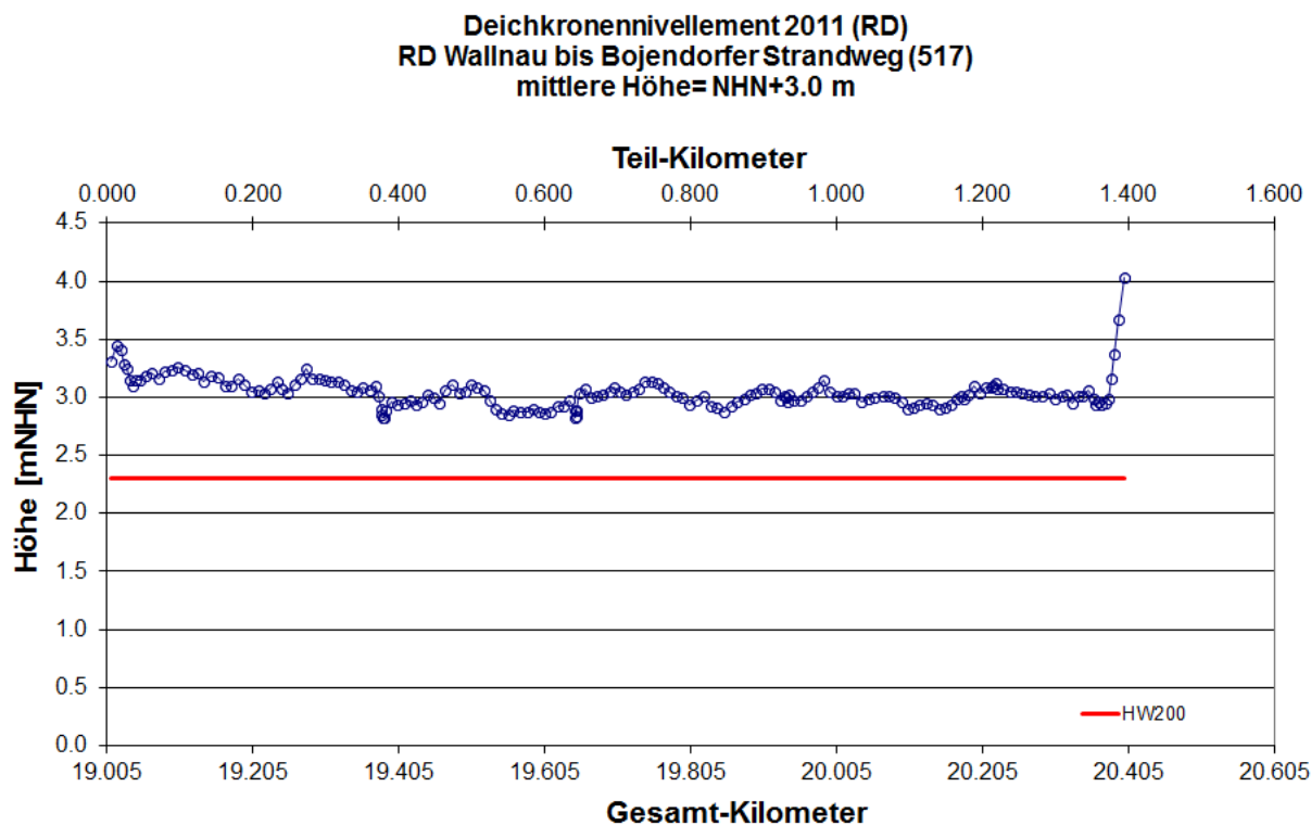
Abb. 137: Längsprofil des Regionaldeiches Flügge bis Wallnau Deichkronennivellement 2011 LKN-SH 2011
