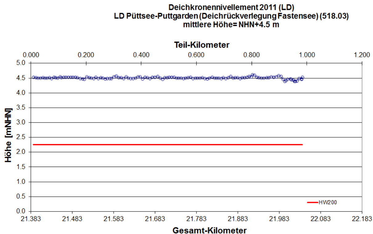
Abb. 174: Längsprofil Landesschutzdeich Püttsee-Puttgarden (Deichrückverlegung Fastensee) Deichkronennivellement 2011 LKN-SH 2011
