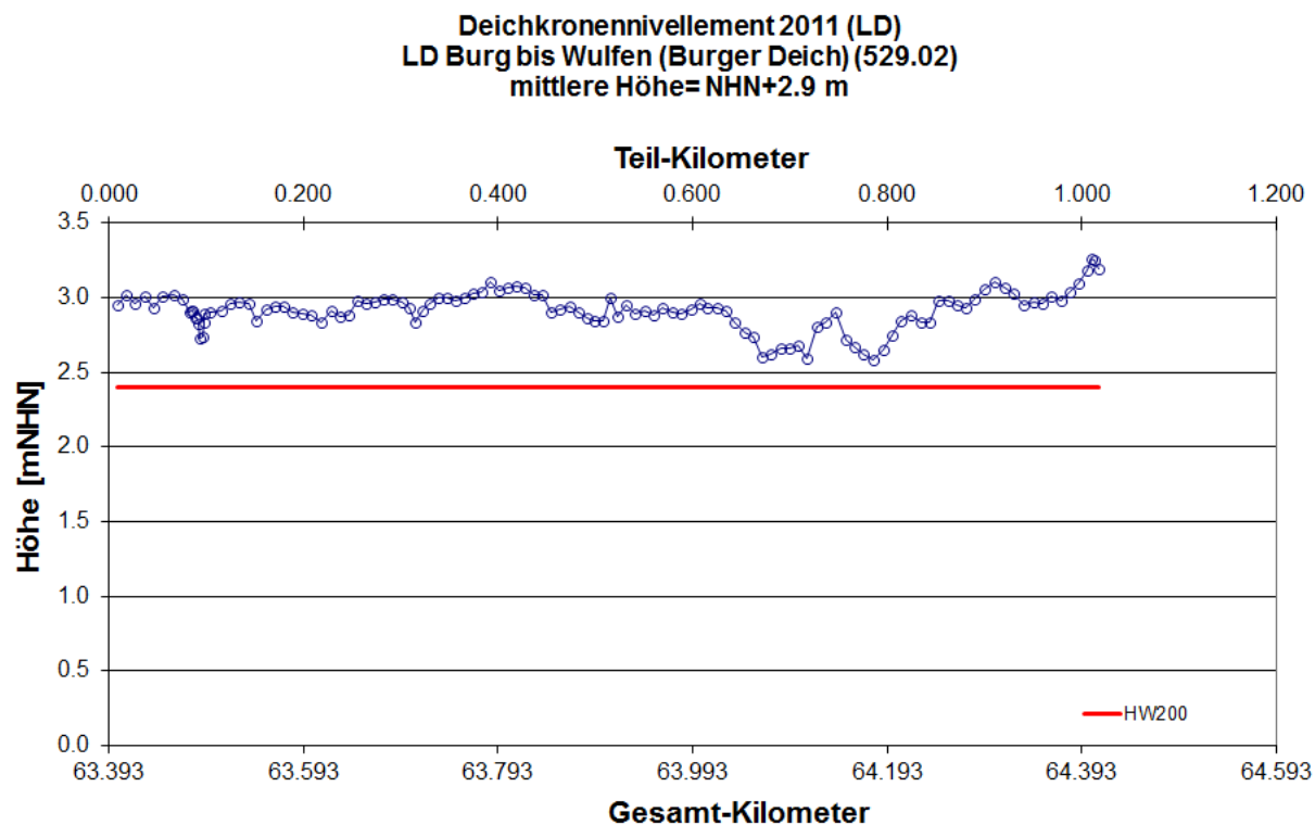
Abb. 300: Längsprofil Landesschutzdeich Burg bis Wulfen (Burger Deich) Deichkronennivellement 2011 LKN-SH 2011
