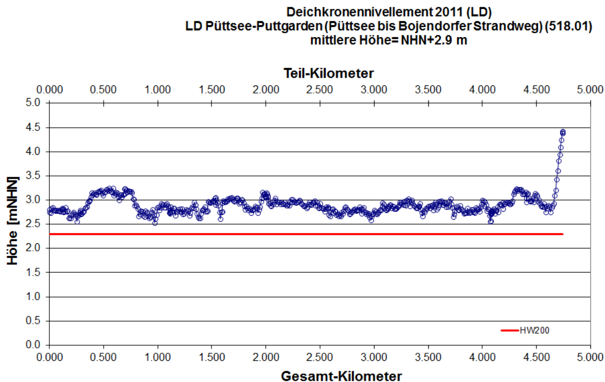
Abb. 150: Längsprofil Landesschutzdeich Püttsee-Puttgarden (Püttsee bis Bojendorfer Strandweg) Deichkronennivellement 2011 LKN-SH 2011
