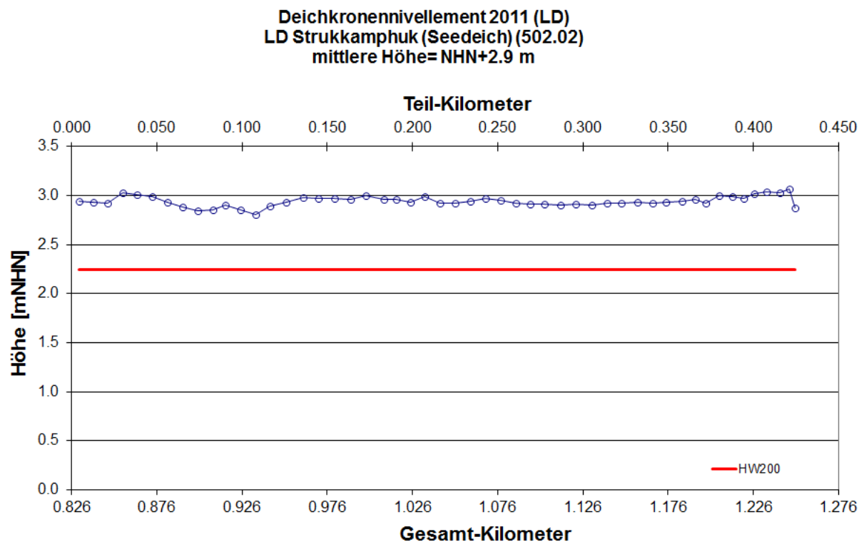
Abb. 9: Längsprofil des Landesschutzdeiches Strukkamphuk (Seedeich) Deichkronennivellement 2011 LKN-SH 2011
