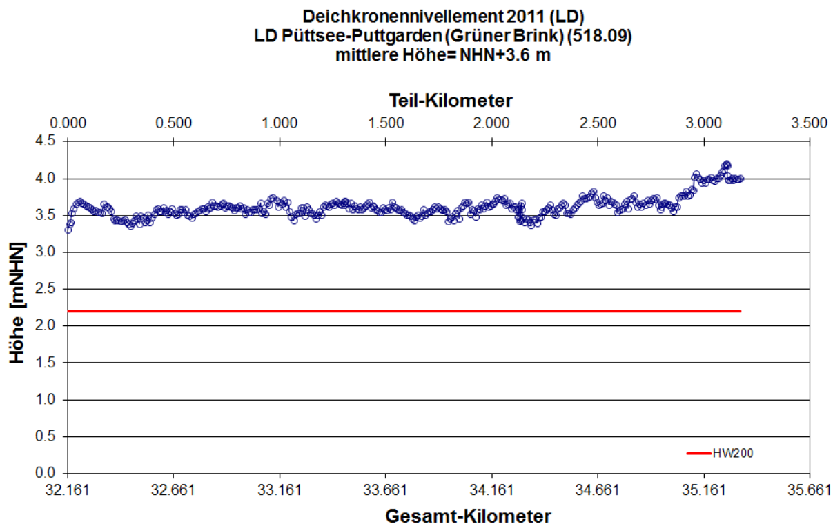
Abb. 242: Längsprofil Landesschutzdeich Püttsee-Puttgarden (Grüner Brink) Deichkronennivellement 2011 LKN-SH 2011
