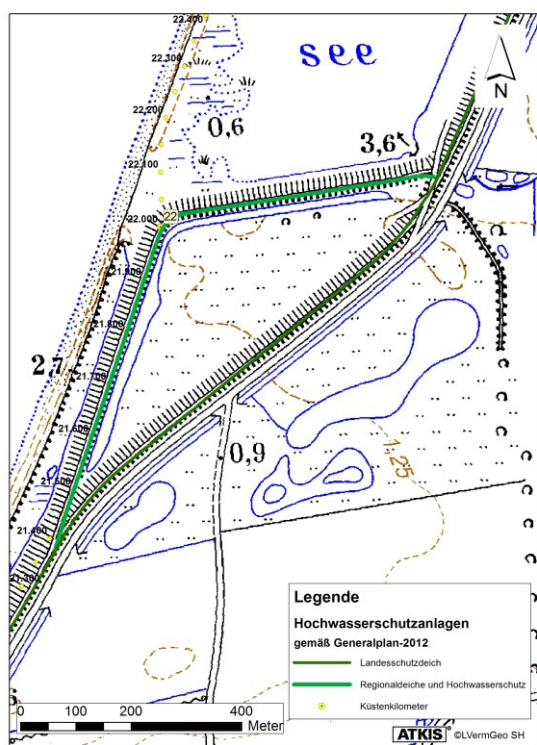
Hochwasserschutz westliches Fehmarn Landesschutzdeich Püttsee-Puttgarden (Deichrückverlegung Fastensee)
