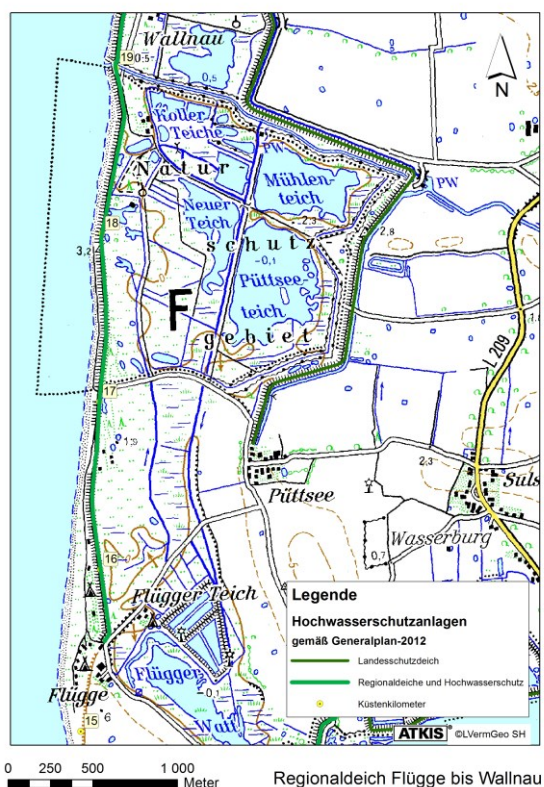
Abb. 122: Lageplan des Regionaldeiches Flügge bis Wallnau LKN-SH 2011
